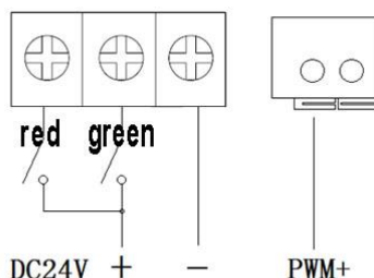
Diagrama cablare
