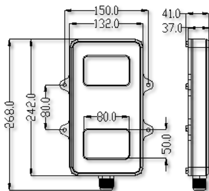
Dimensiuni (mm)
